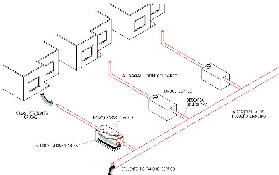
Figura 1. Componentes de redes de alcantarillado sin arrastre de sólidos.
