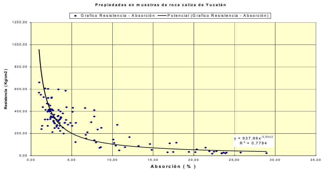
Figura 9. Correlación Resistencia - Absorción
