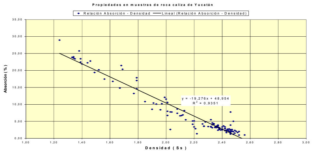
Figura 10. Correlación Absorción - Densidad
