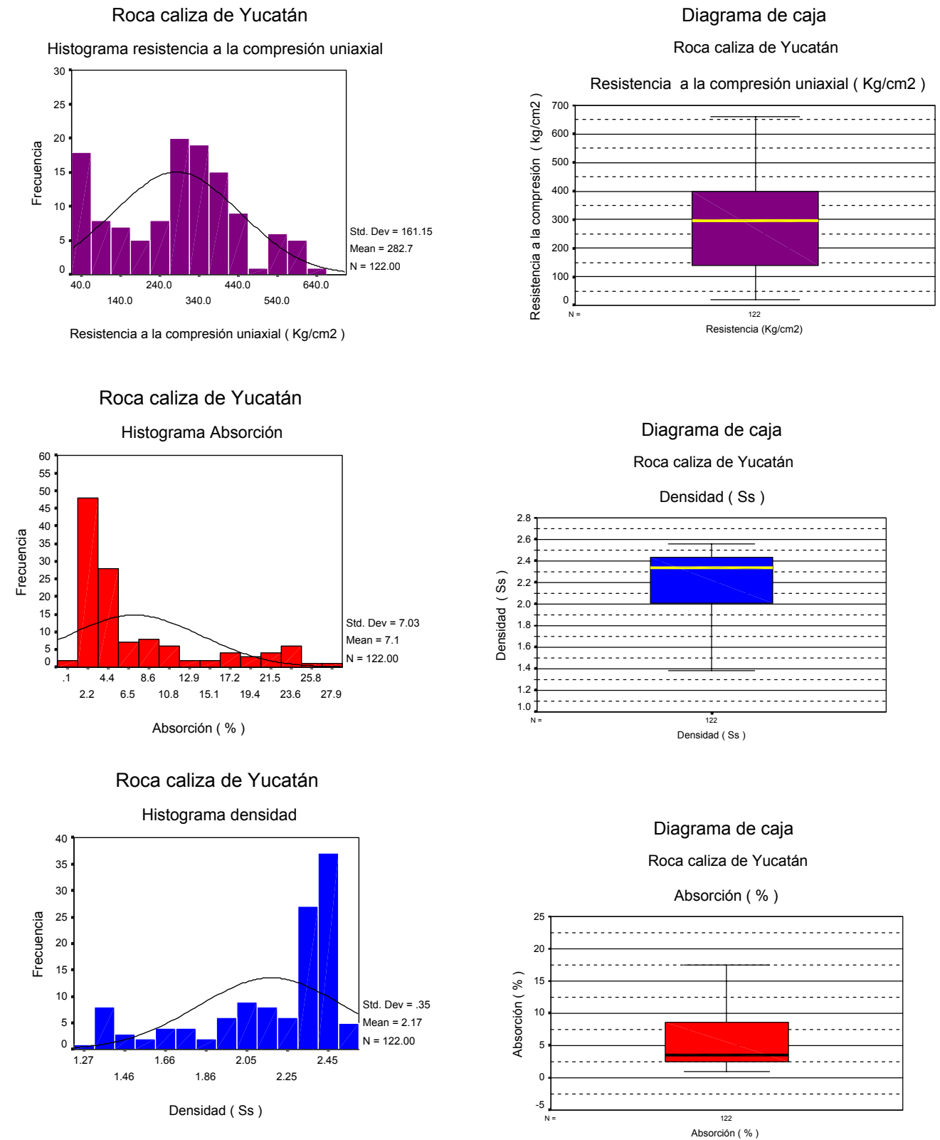
Figura 7. Histogramas y diagramas de caja de las pruebas realizadas
