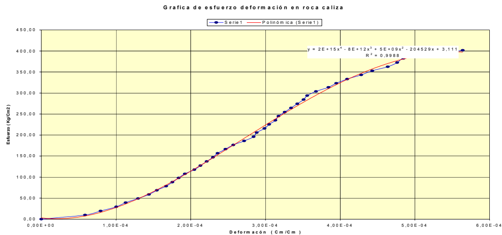
Figura 12. Correlación Esfuerzo – Deformación unitaria.
